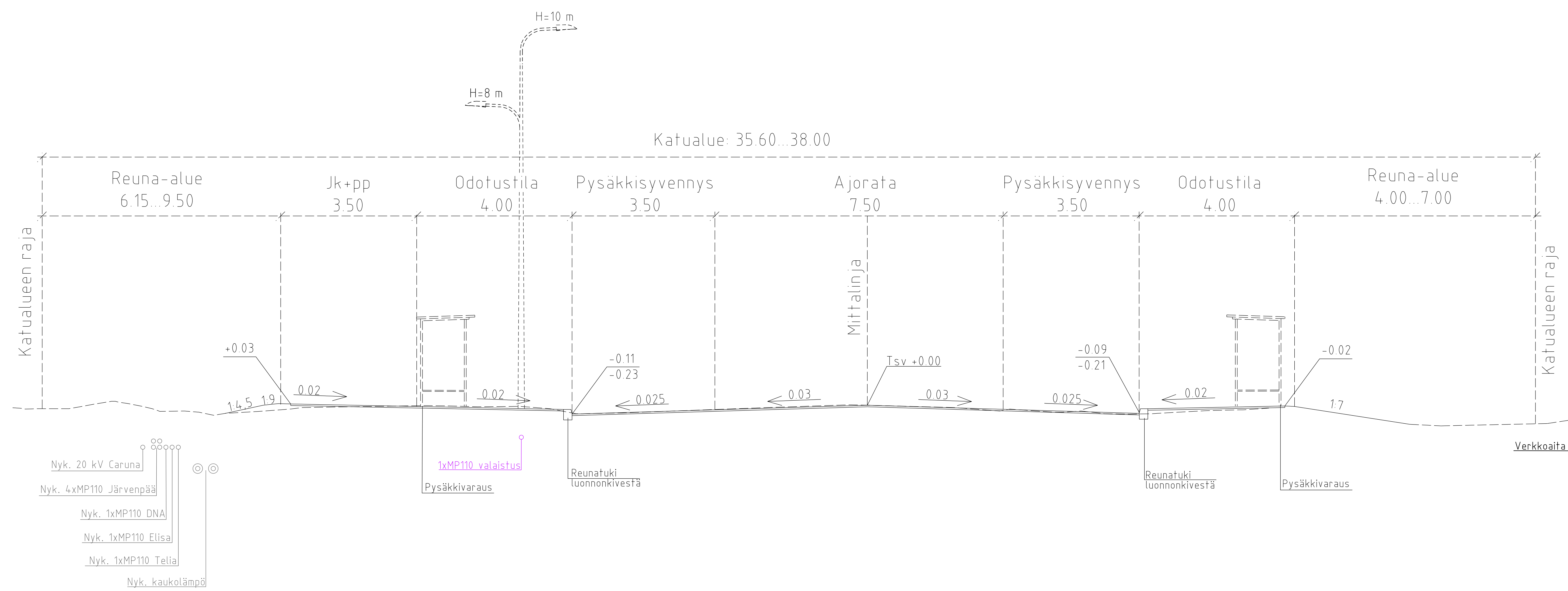
Tyypipoikkileikkaus plv 370-422 (pl 400) 1:100
